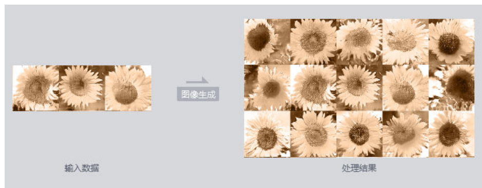
图 3-4 StyleGan 算子
